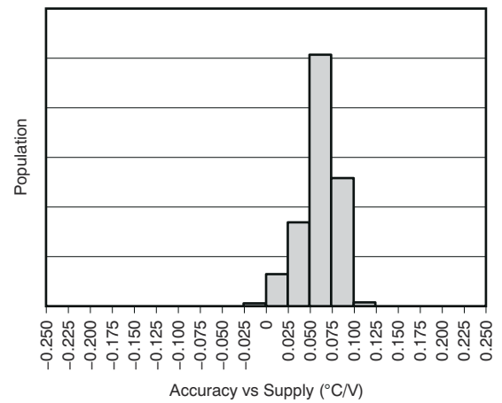
图 6-3. 精度与电源间的关系
