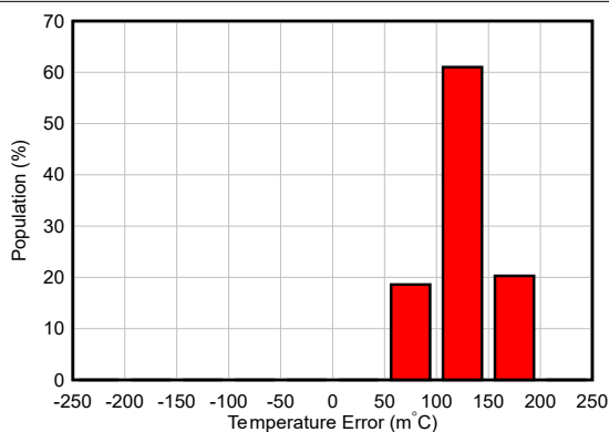
图 6-19. 25°C 时的温度误差
