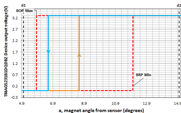
图 9-6. 阈值
