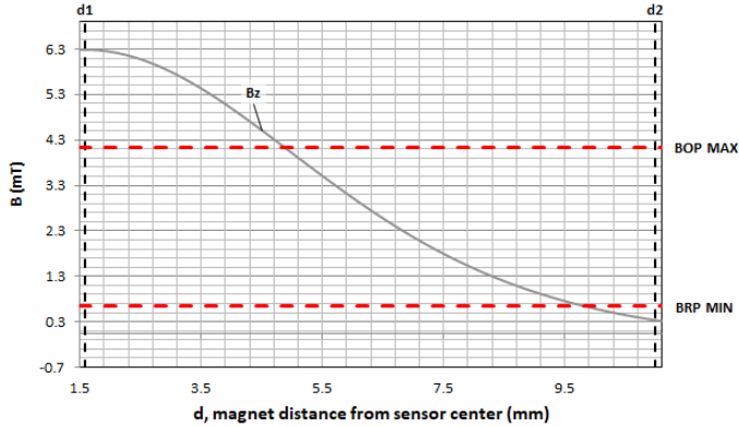
图 9-12. B 场假设
