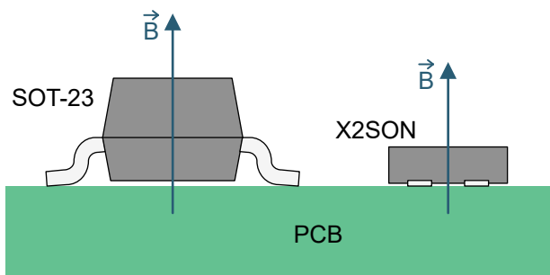
图 8-1. 灵敏度方向
