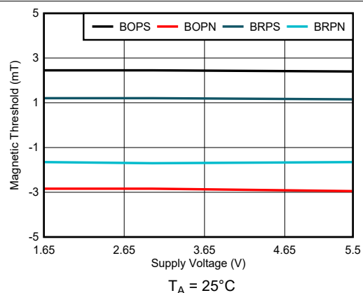
图 7-4. 2.85mT 阈值与电源电压之间的关系
