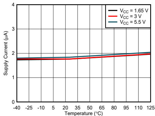
图 7-8. I_{CC} 与温度之间的关系
