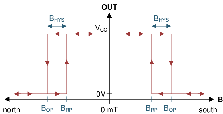
图 8-3. 全极功能
