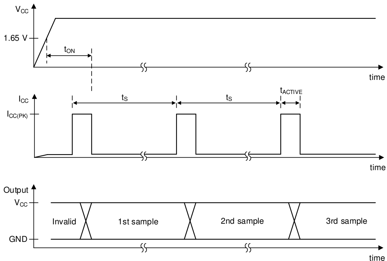
图 8-5. 时序图
