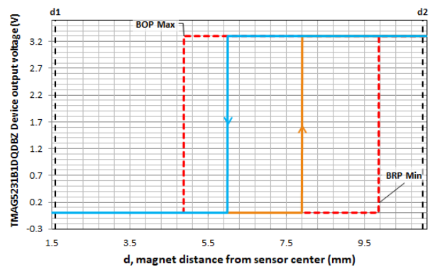
图 9-13. 阈值
