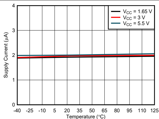
图 7-10. I_{CC} 与温度之间的关系
