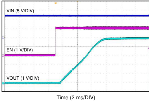
V_{IN} = 12\text{ V} V_{OUT} = 5\text{ V} I_{OUT} = 2\text{ A} 图 7-2. 由 EN 启动
