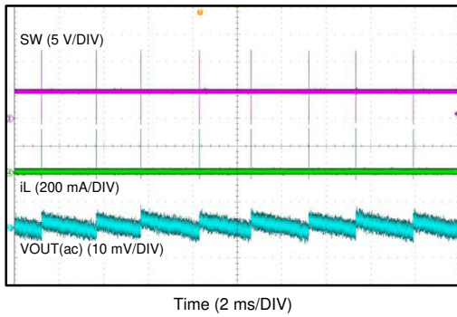
V_{IN} = 12\text{ V} V_{OUT} = 5\text{ V} I_{OUT} = 0\text{ A} 图 7-4. 睡眠模式
