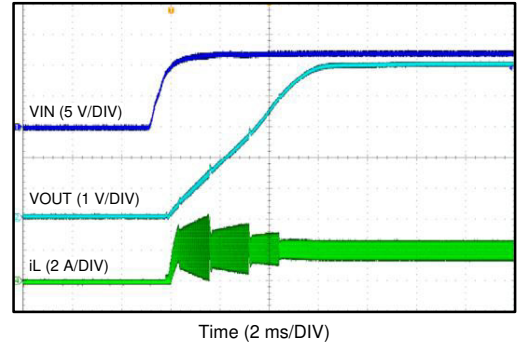
V_{IN} = 12\text{ V} V_{OUT} = 5\text{ V} I_{OUT} = 2\text{ A} 图 7-3. 由 V_{IN} 启动
