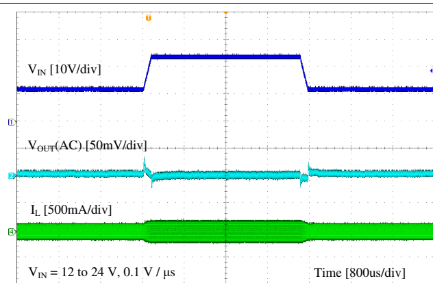
图 8-8. Line Transient
