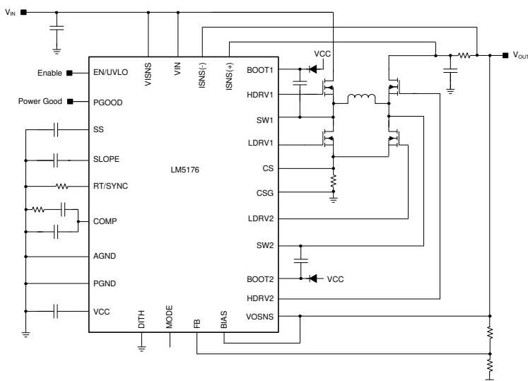
简化原理图
