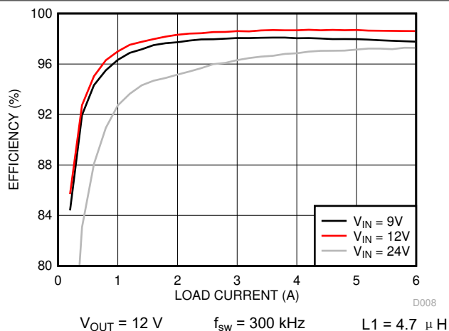
图 6-2. Efficiency vs Load
