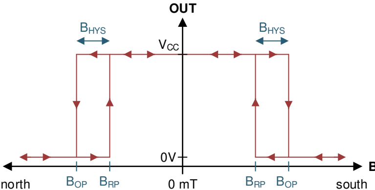
图 7-3. 全极功能
