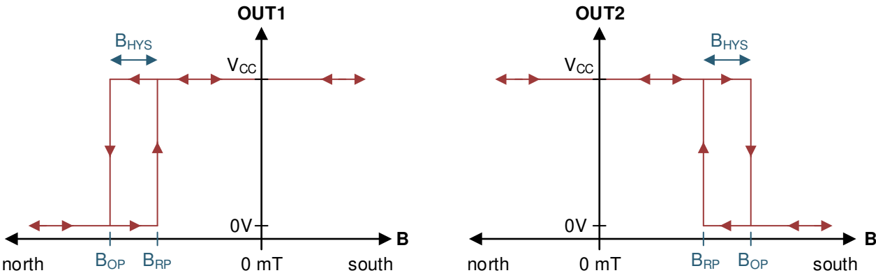
图 7-4. 单极功能
