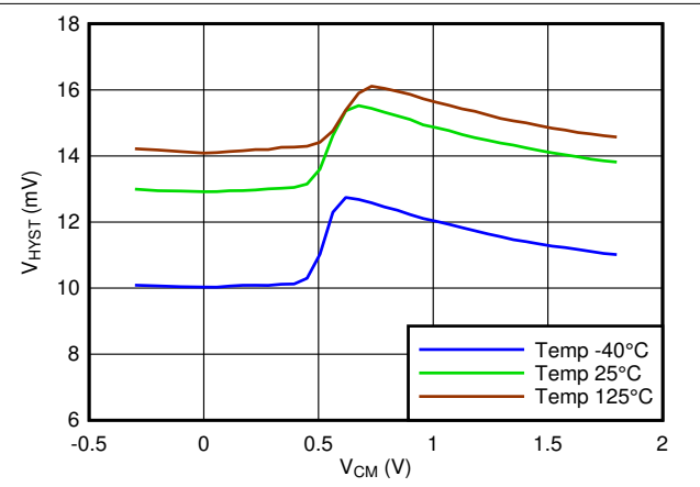
图 5-12. Hysteresis vs V_{CM}
