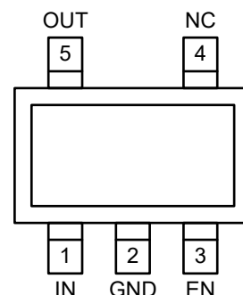
CJ6101BxxM SOT-23-5L
