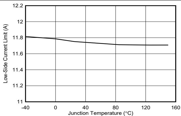
图 5-8. 低侧谷值电流限制与温度间的关系
