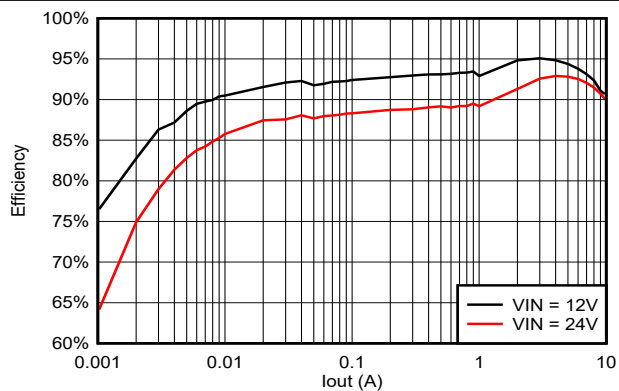
图 5-12. 效率, V_{out} = 3.3V , F_{sw} = 500kHz
