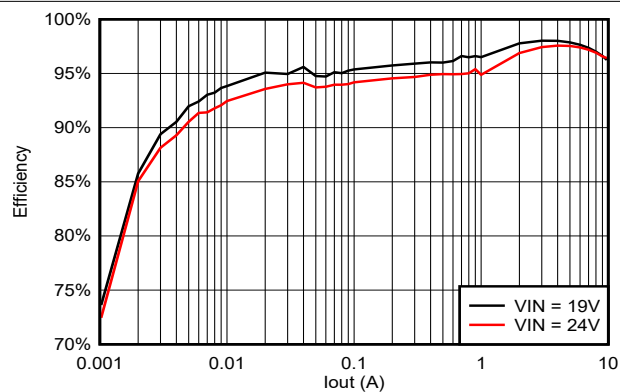
图 5-14. 效率, V_{out} = 12V , F_{sw} = 500kHz
