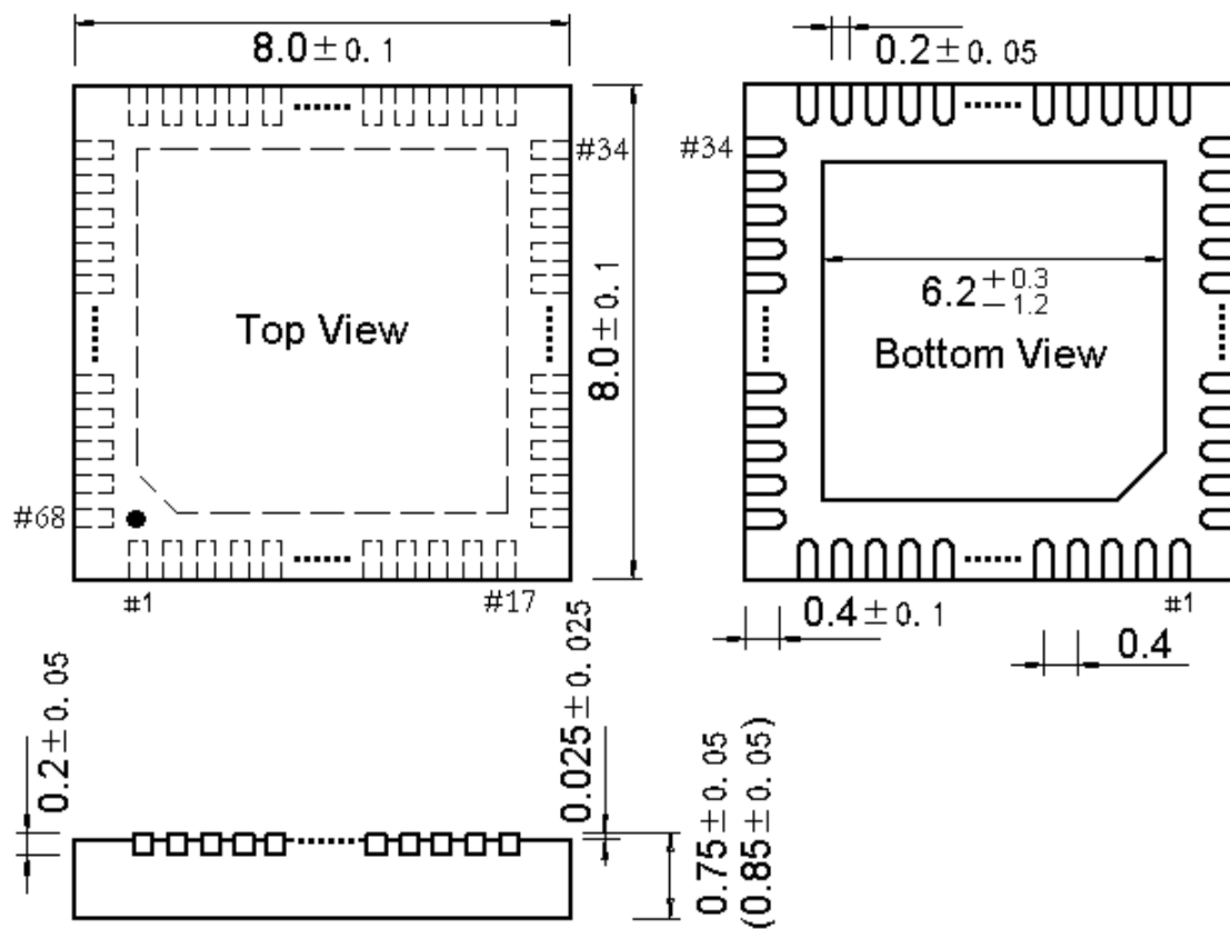
图 5-6 QFN68 封装
