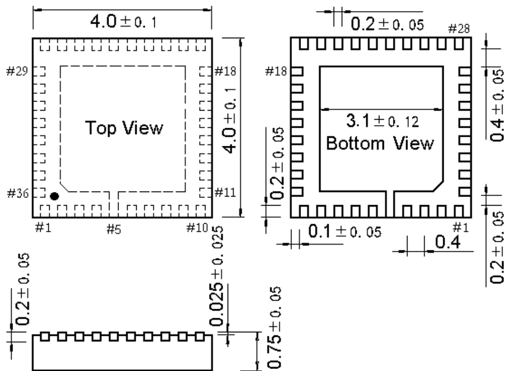
图 5-3 QFN36C4 封装
