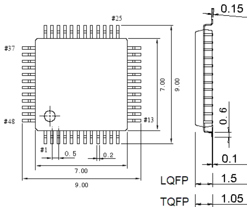
图 5-4 LQFP48 封装
