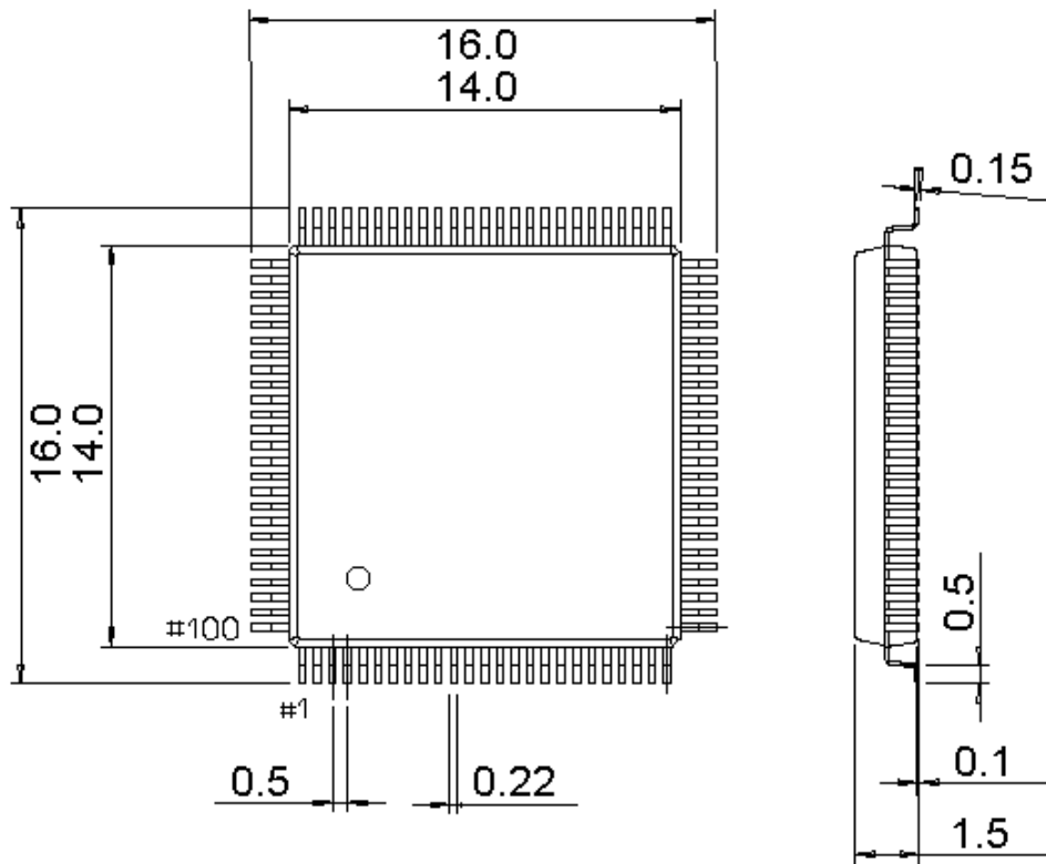
图 5-7 LQFP100 封装
