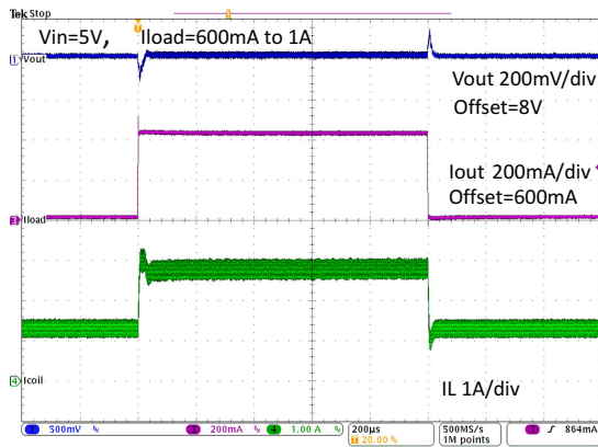
图 9-20. Load Transient
