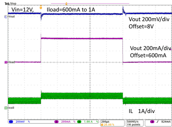
图 9-21. Load Transient
