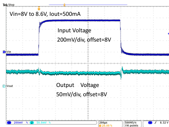
图 9-22. Line Transient
