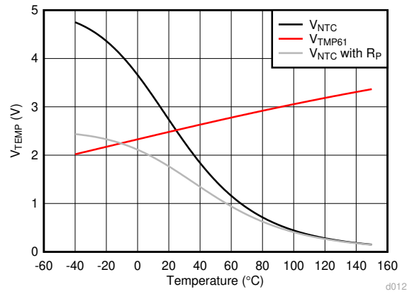
图 8-9. 带和不带线性电阻的 NTC 与 TMP61 温度电压
