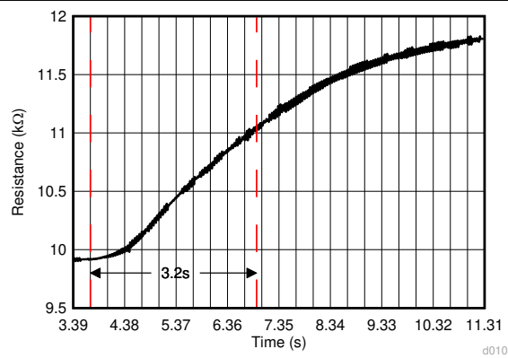
图 6-7. 阶跃响应
