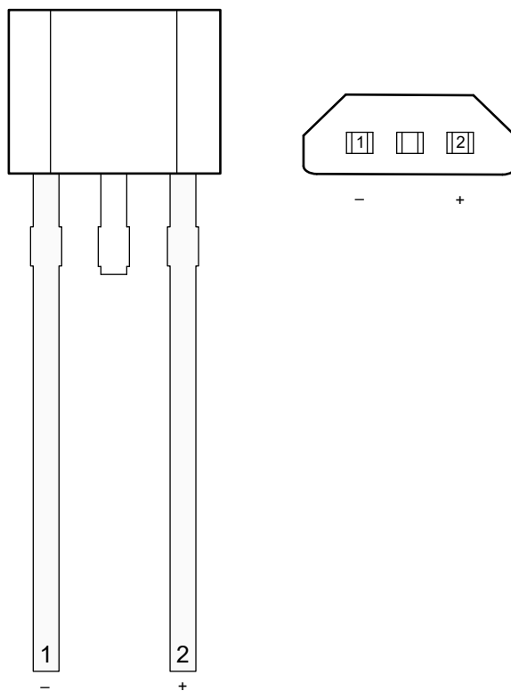
图 5-3. LPG 封装 2 引脚 TO-92S 前视图、底视图
