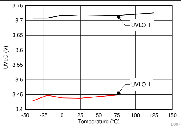
图 5-12. UVLO 阈值
