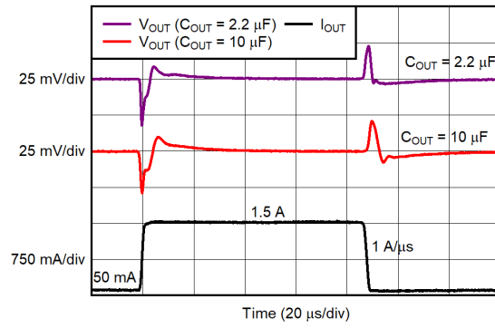
图 5-36. 输出负载瞬态响应
