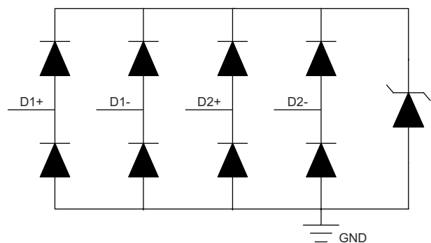
TPD4E05U06 功能方框图
