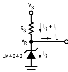
图 8-1. 并联稳压器原理图
