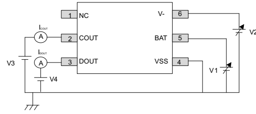
图 7-6. Test Circuit 4
