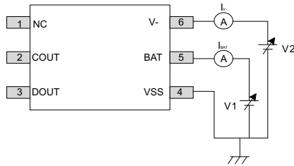
图 7-5. Test Circuit 3
