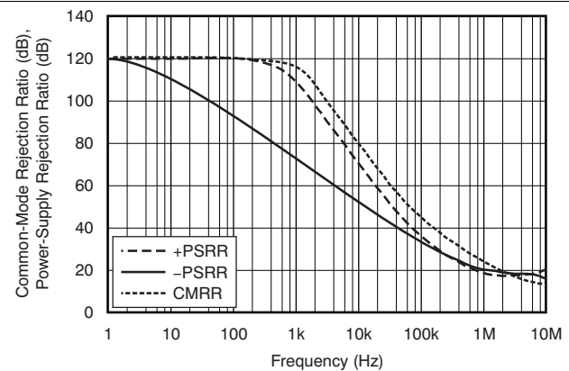
图 6. CMRR 和 PSRR 与频率间的关系 (以输入为参考)
