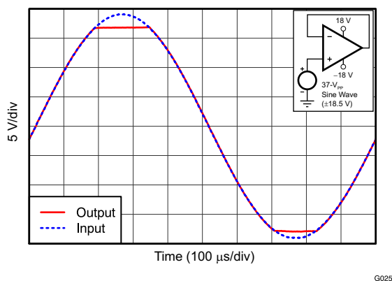
图 26. 无相位反转
