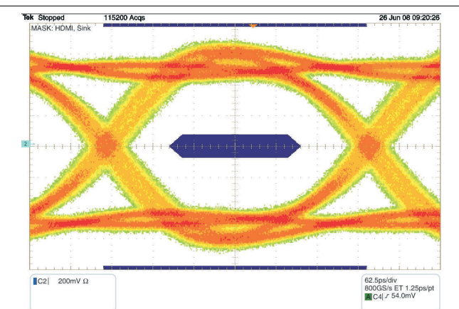
图 7-3. 含有 TPD8S009 的眼图 ( 2.5Gbps 数据速率 )
