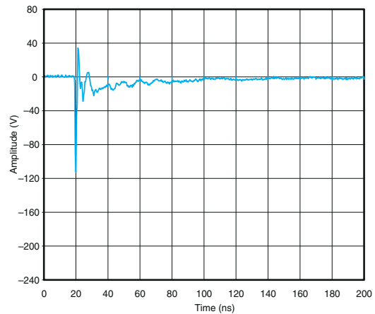
图 5-4. 图 3.IEC 钳位波形 (-8kV 接触)
