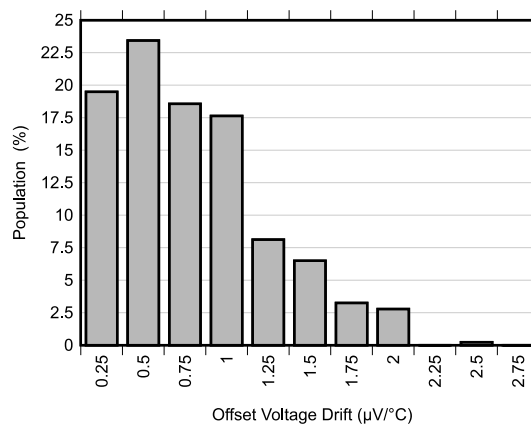
图 6-2. 失调电压漂移分布
