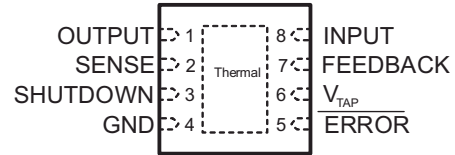
图 4-2. DRG 封装, 8 引脚 WSON (带外露散热焊盘) (顶视图)
