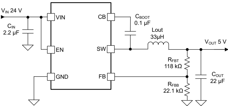
图 8-1. 应用电路
