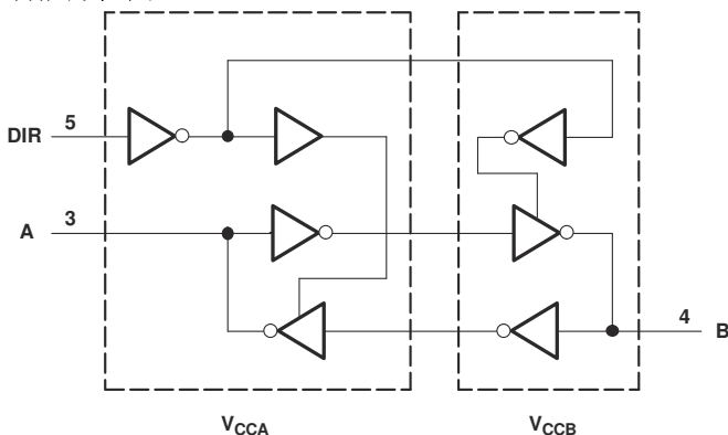
功能方框图
