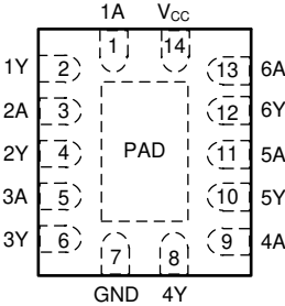
图 4-2. SN74ACT14 BQA 封装, 14 引脚 WQFN (顶视图)
