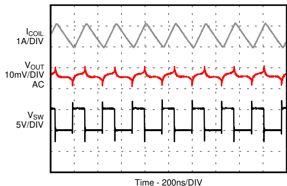
图 8-27. PWM Operation
