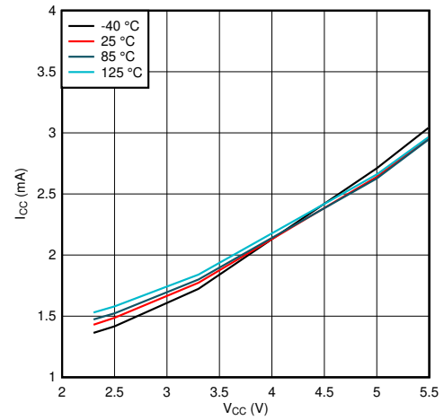
图 6-2. I_{CC} vs V_{CC}
