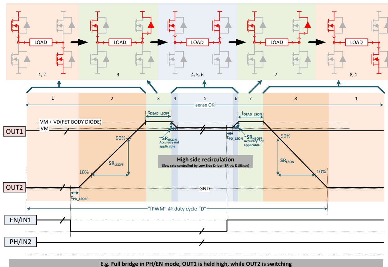
图 7-2. 具有高侧再循环的 H 桥的输出开关瞬变
