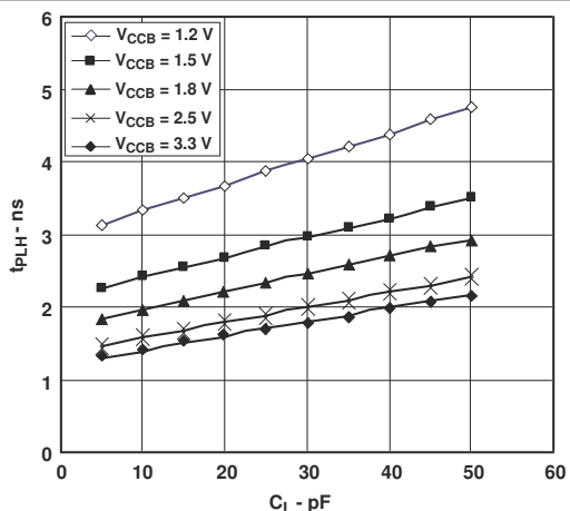
图 5-7. 高电平到低电平 (A 到 B) 的典型传播延迟与负载电容间的关系 T_A = 25^\circ\text{C} , V_{CCA} = 2.5V
