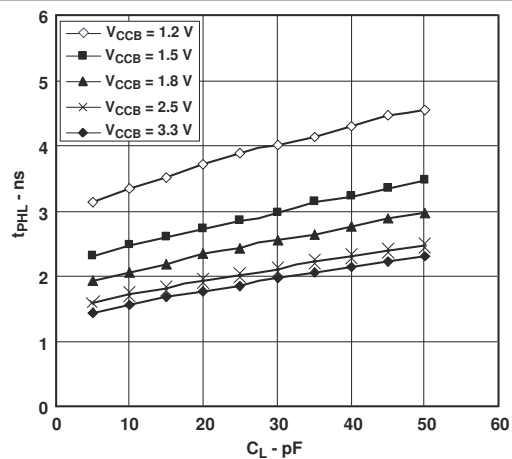
图 5-8. 低电平到高电平 (A 到 B) 的典型传播延迟与负载电容间的关系 T_A = 25^\circ\text{C} , V_{CCA} = 2.5V
