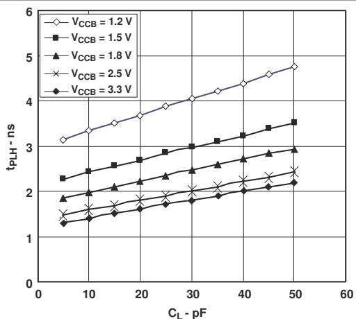
图 5-9. 高电平到低电平 (A 到 B) 的典型传播延迟与负载电容间的关系 T_A = 25^\circ\text{C} , V_{CCA} = 3.3V
