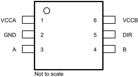
图 4-3. DRL 封装，6 引脚 SOT-5X3 ( 顶视图 )
