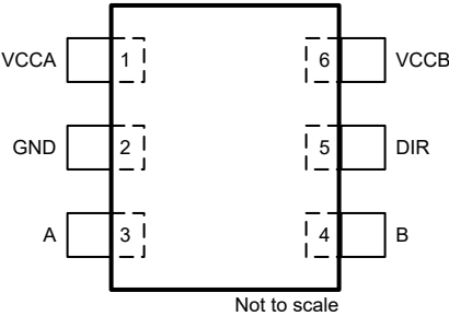
图 4-1. DBV 封装， 6 引脚 SOT-23 ( 顶视图 )
