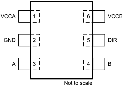
图 4-2. DCK 封装，6 引脚 SOT-SC70 ( 顶视图 )
