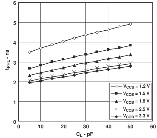
图 5-4. 低电平到高电平 (A 到 B) 的典型传播延迟与负载电容间的关系 T_A = 25^\circ\text{C} , V_{CCA} = 1.5\text{V}
