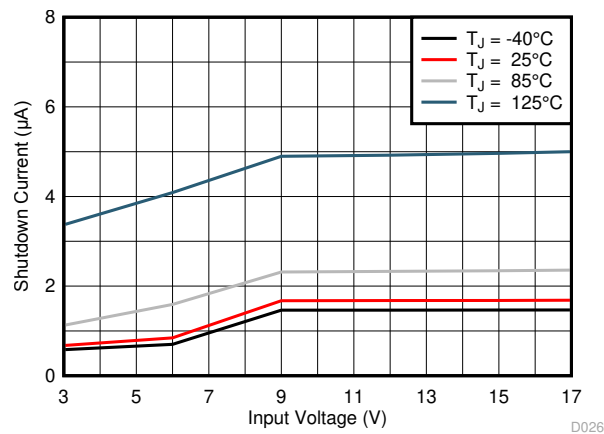
图 6-3. 关断电流
