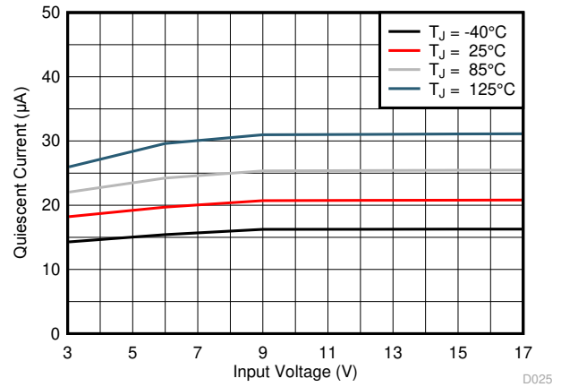
图 6-2. 静态电流
