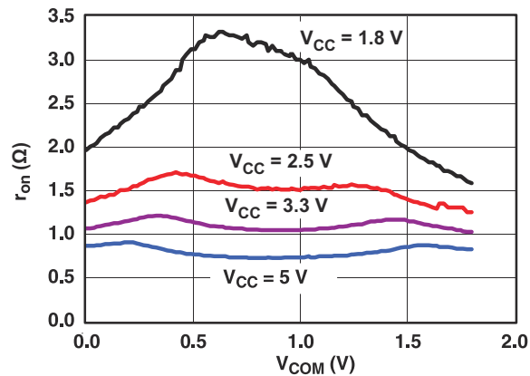
图 9-2. R_{on} vs V_{COM}
