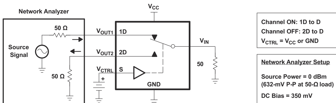
图 6-3. Crosstalk ( X_{TALK} )
