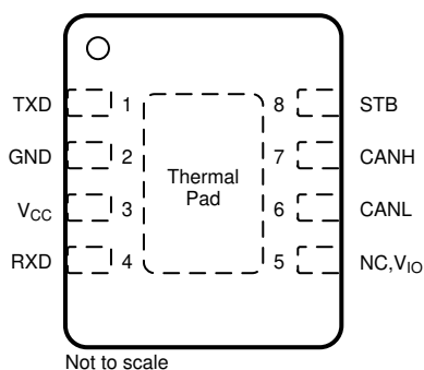
图 5-3. DRB Package, 8-Pin VSON (Top View)
