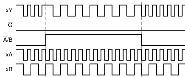
图 7-2. 应用时序图
