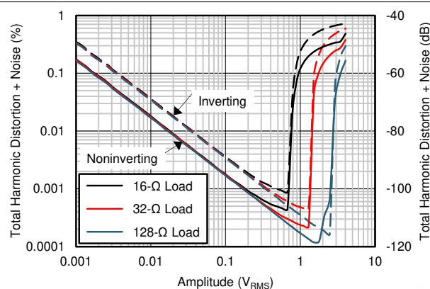
图 7-16. THD+N vs Output Amplitude
