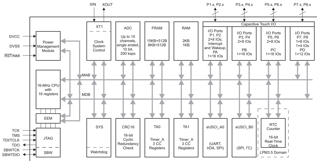
图 1-1. 功能框图
