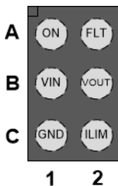
图 6-1. TPS22950x WCSP - 6 Top View
