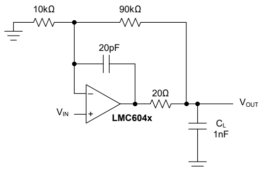
图 6-2. LMC604x 非反向增益 10 放大器，在经过补偿后可处理电容负载
