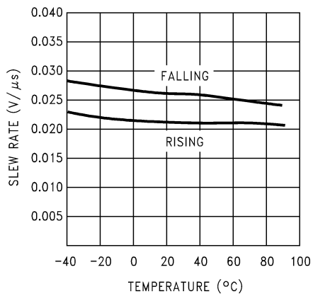
图 5-19. 非反向转换率与温度
