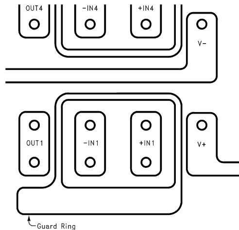
图 6-14. PCB 布局中的防护环示例
