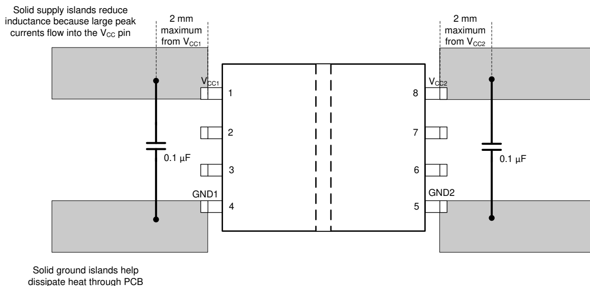
图 11-1. Layout Example
