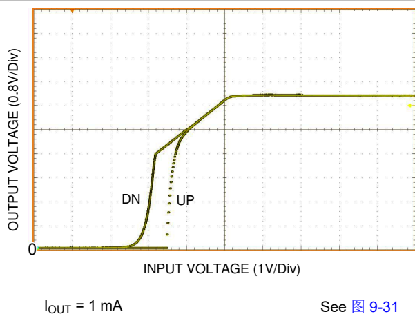
图 7-5. UVLO Thresholds
