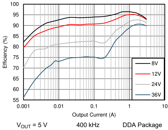
图 9-7. Efficiency
