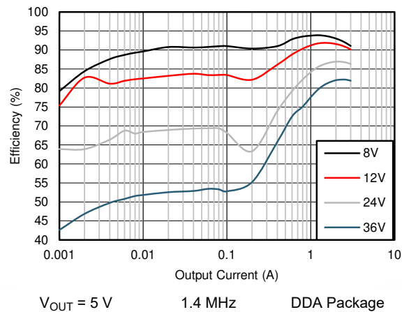
图 9-9. Efficiency
