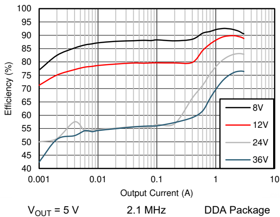
图 9-11. Efficiency
