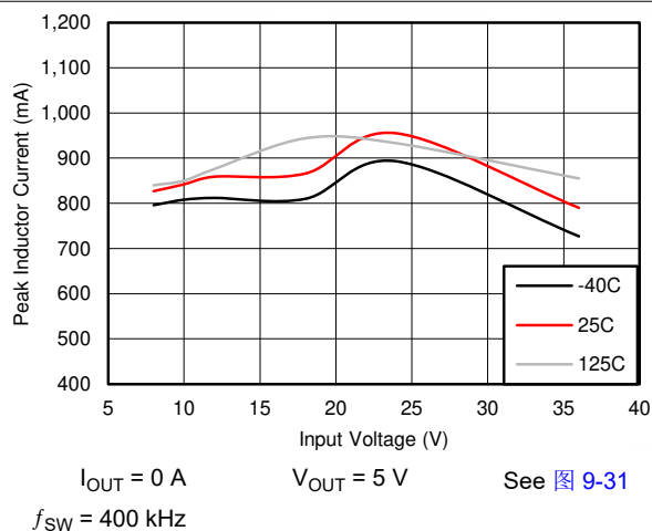
图 7-6. I_{PEAK-MIN}
