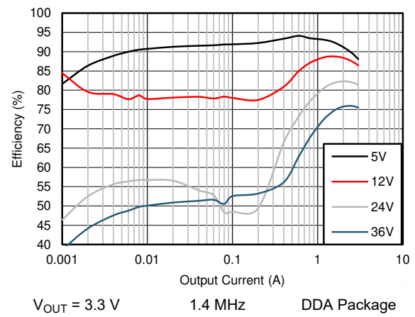
图 9-10. Efficiency
