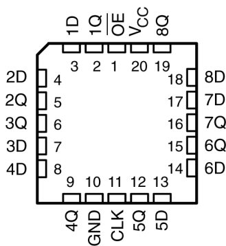
图 3-2. SN54ACT374 FK Package (Top View)
