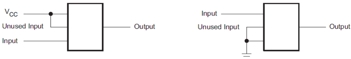
图 7-1. Layout Example
