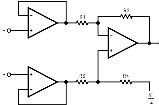
图 9-5. 三级运算放大器仪表放大器
