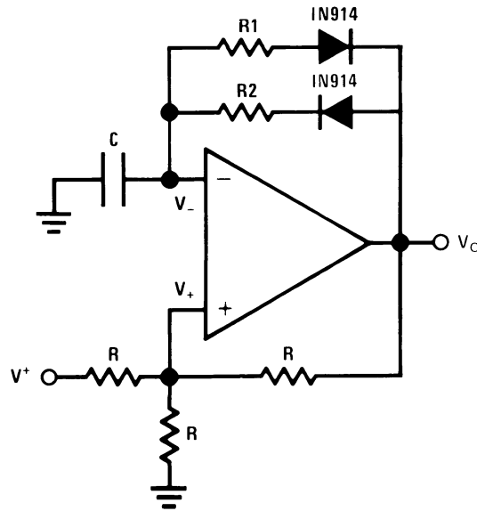
图 9-11. 脉冲发生器
