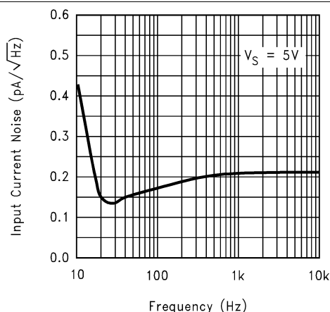
图 7-10. 输入电流噪声与频率之间的关系
