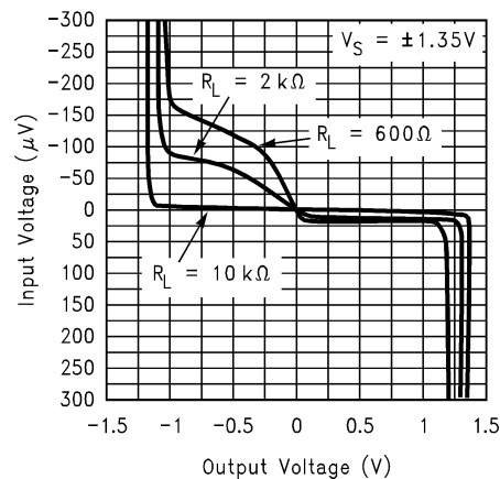
图 7-18. 输入电压与输出电压之间的关系
