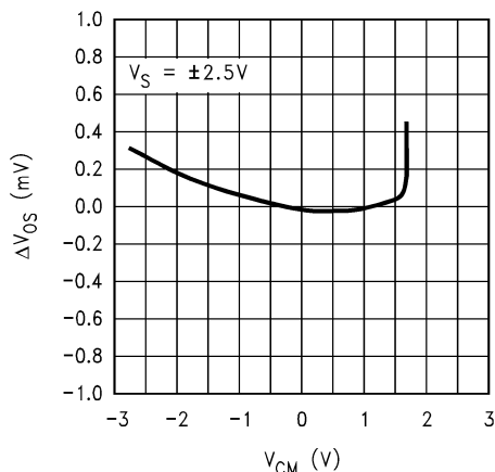
图 7-17. \Delta V_{OS} 与 CMR 之间的关系
