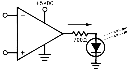
图 9-18. LED 驱动器
