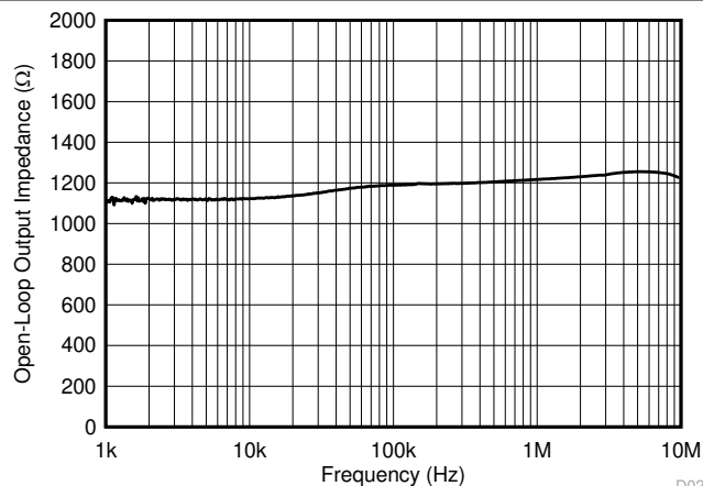
图 7-44. 开环输出阻抗与频率之间的关系 (LM3xx-N)
