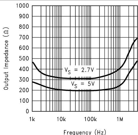
图 7-43. 开环输出阻抗与频率之间的关系
