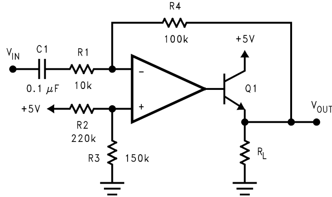
图 9-17. 功率放大器
