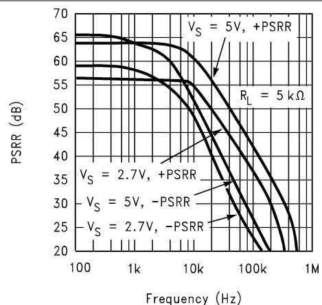
图 7-12. PSRR 与频率之间的关系
