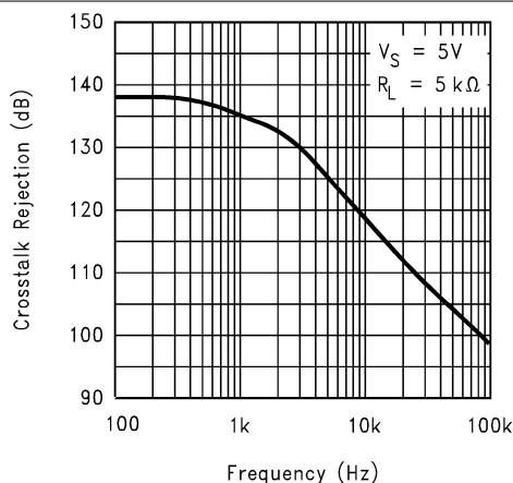
图 7-11. 串扰抑制与频率之间的关系
