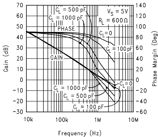
图 7-23. 增益和相位与容性负载之间的关系
