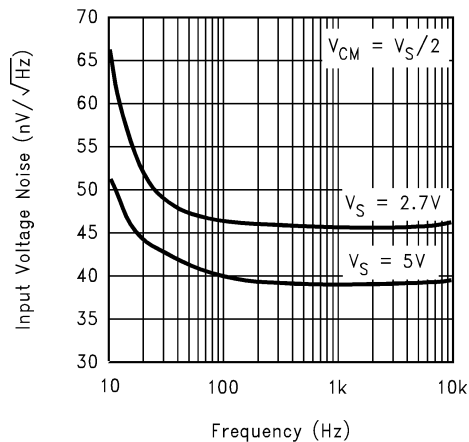
图 7-8. 输入电压噪声与频率之间的关系
