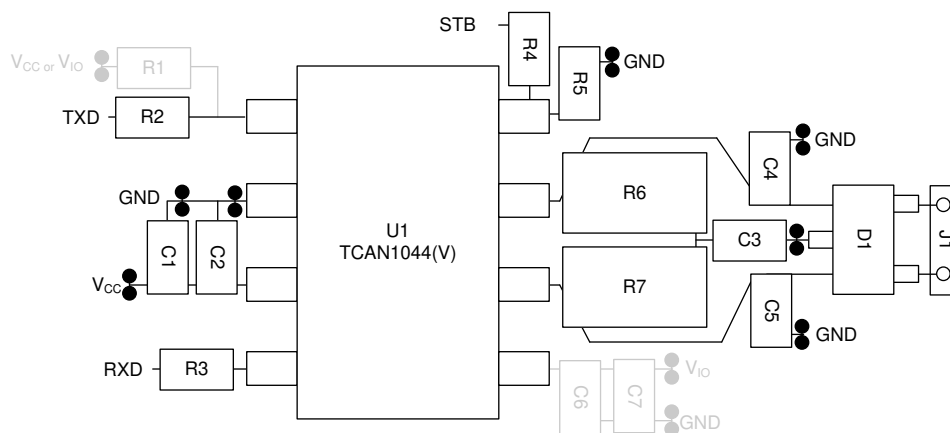
图 9-7. Layout Example
