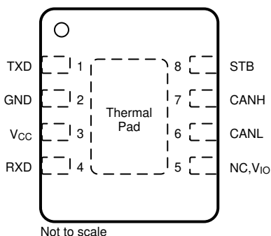
图 5-3. DRB Package, 8-Pin VSON (Top View)
