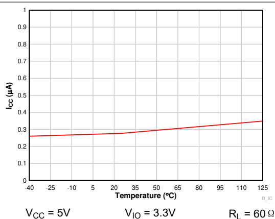
图 6-3. I_{CC} Standby vs Temperature
