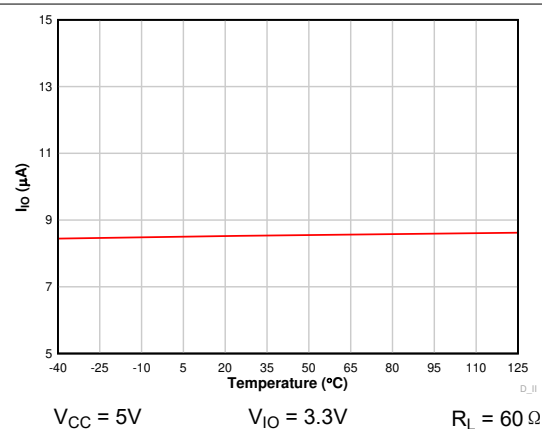
图 6-4. I_{IO} Standby vs Temperature
