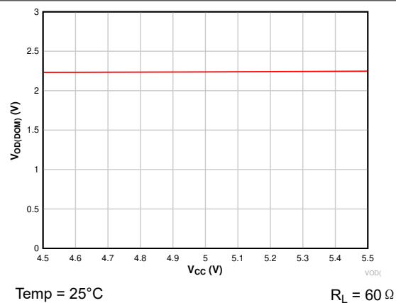
图 6-2. V_{OD(DOM)} vs V_{CC}
