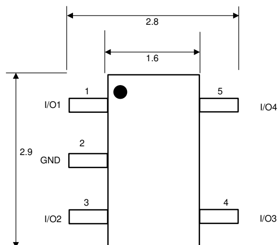
图 4-2. ESDS304 DBV Package, 5-Pin SOT23 (Top View)
