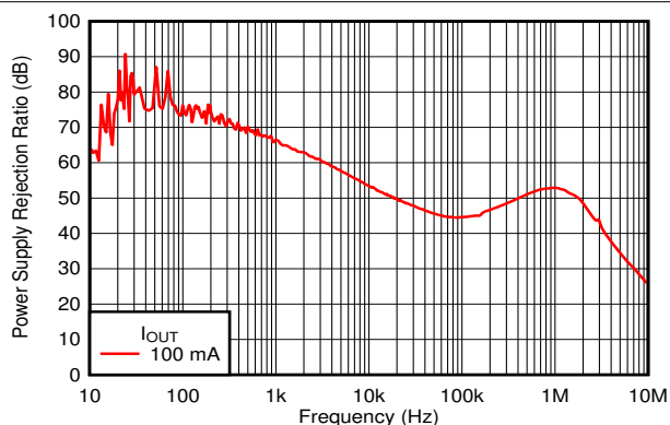
图 9-4. PSRR Performance
