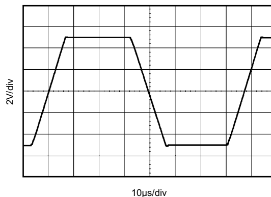
图 6-20. 大信号阶跃响应
