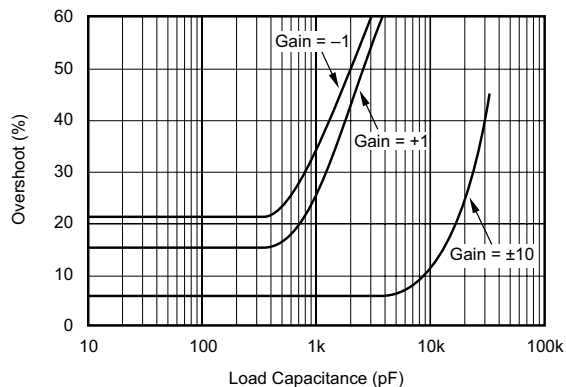
图 6-19. 小信号过冲与负载电容间的关系
