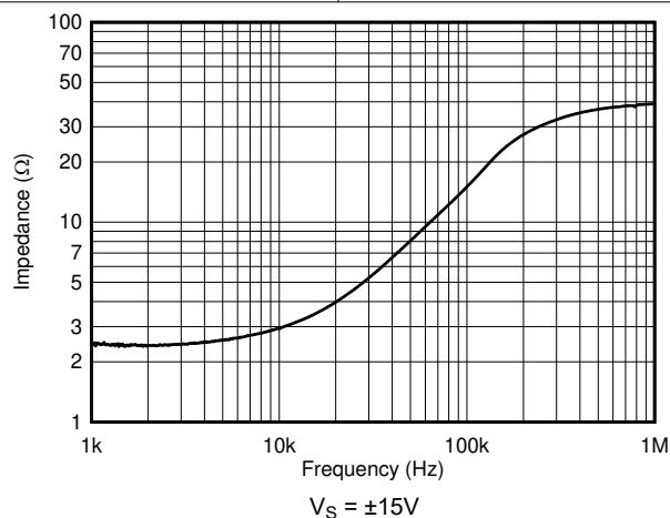
图 6-23. 开环输出阻抗
