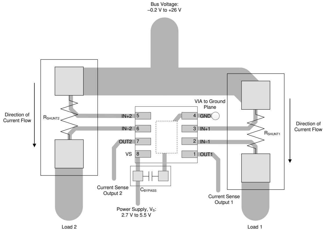
图 9-9. 双通道推荐布局 (WSN)
