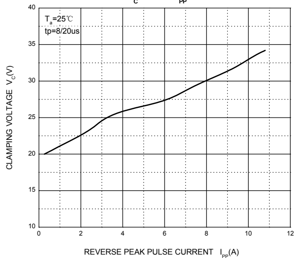
V_C — I_{PP}
