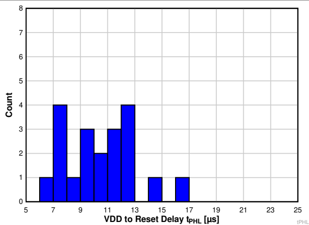
图 6-15. TPS3823A-33 器件在 -40°C 时的 VDD 至复位延时直方图 (单位数 = 20)
