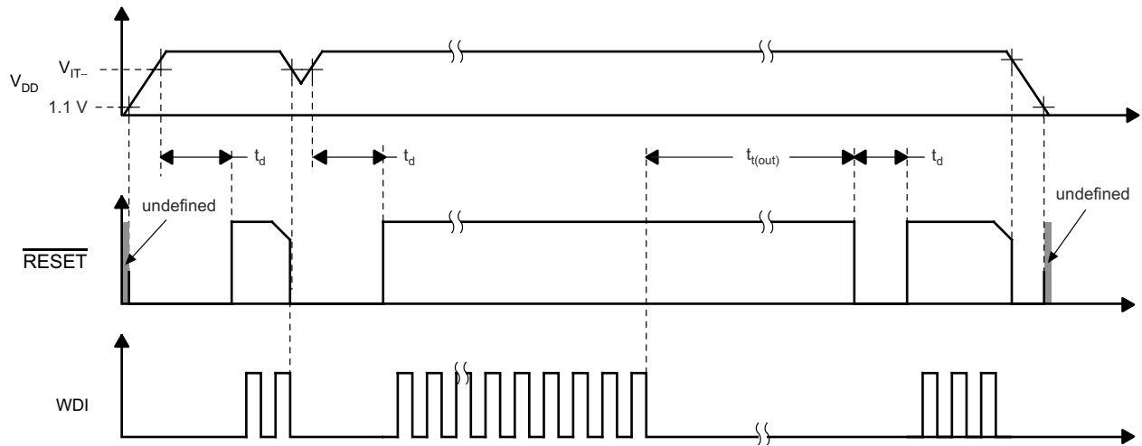
图 6-1. 时序图
