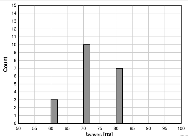
图 6-25. TPS3823A-33 器件在 25°C 时的 WDI 脉宽直方图 (单位数 = 20)
