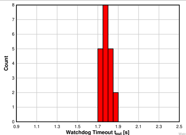
图 6-14. TPS3823A-33 器件在 125°C 时的看门狗超时直方图 (单位数 = 20)
