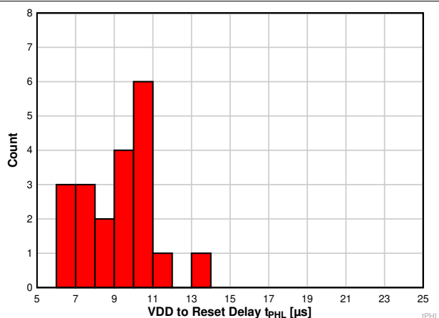
图 6-17. TPS3823A-33 器件在 125°C 时的 VDD 至复位延时直方图 (单位数 = 20)
