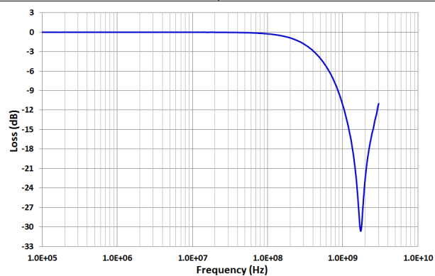
图 5-9. Insertion Loss
