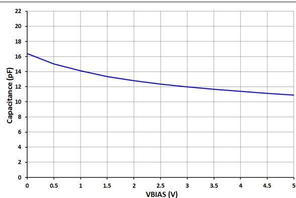
图 5-8. Pin Capacitance Across V_{BIAS}
