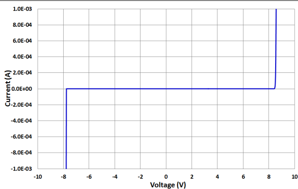
图 5-5. IV Curve
