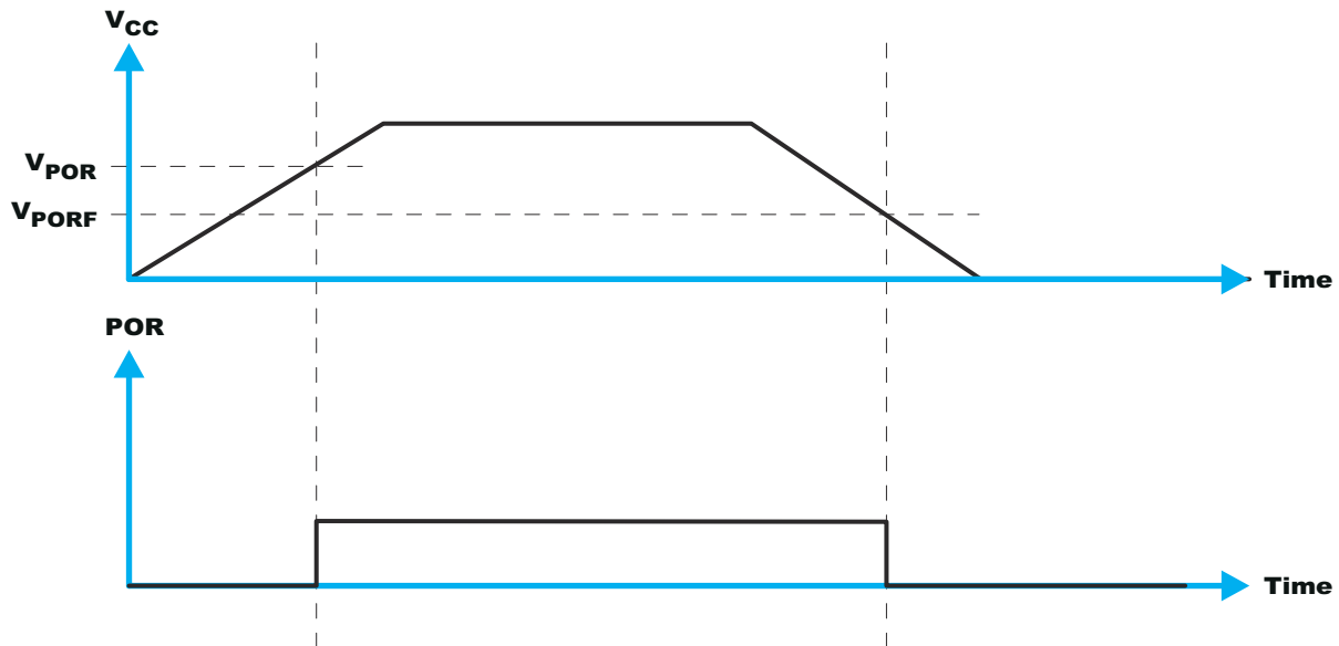
图 10-4. V_{POR}
